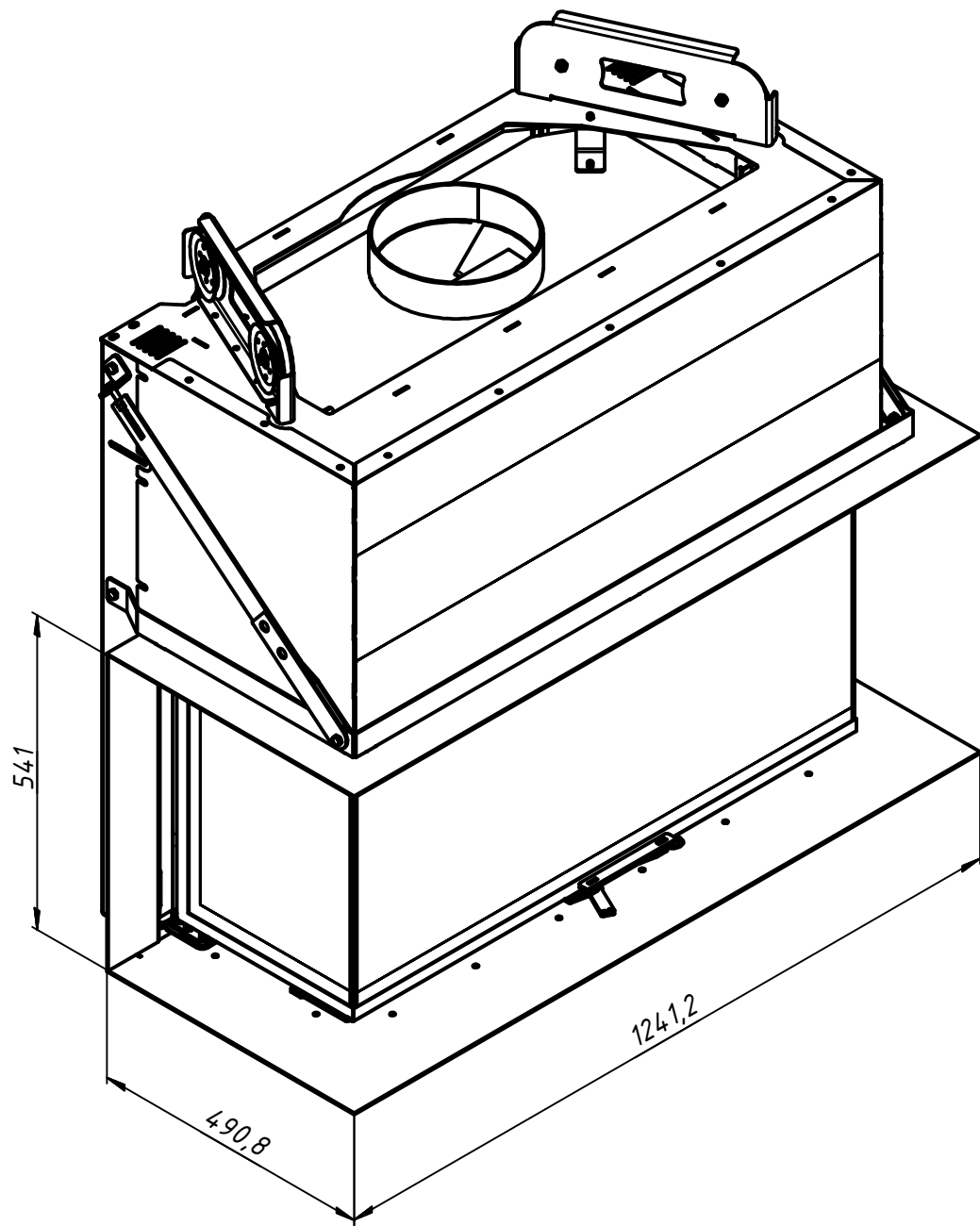
Монтажна рама 1,5мм 1x90
